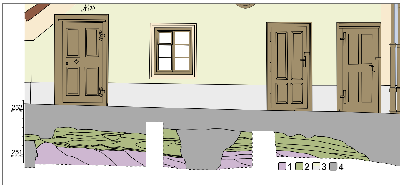
Obr. 13. Praha 1-Hrad, Zlatá ulička. Severní řez pod čelní stěnou domu čp. 23 ve Zlaté uličce: 1 – souvrství z období před rudolfínskou přestavbou; 2 – souvrství z rudolfínské přestavby narušené mladšími zásahy; 3 – nadzemní zdivo čp. 23; 4 – hradební a základové zdivo pod úrovní dnešní komunikace (kresba J. Matíášek, 2017).
