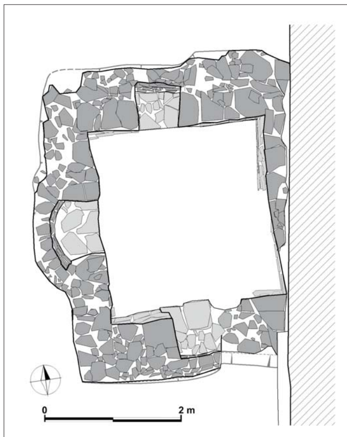
Obr. 7. Praha 1-Staré Město, čp. 190, Klementinum. Půdorys břídicové jímký (kresba J. Hlavatý a N. Hladíková Trachtová, 2011).
