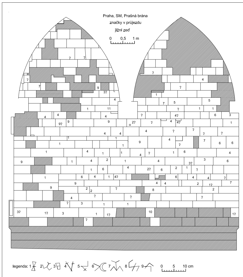
Obr. 6. Praha 1-Staré Město, Prašná brána, jižní stěna průjezdu. Výkres spárořezu s vyznačením pozic nalezených značek. Měřítka výkresu 1:50, měřítka legendy (překreslených značek) 1:5. Otazníkem jsou naznačeny pozice pravděpodobných kamenických značek, jejichž podoba není při dokumentaci z terénu rozpoznatelná. Šrafovou vymezeny plochy novodobě vyměněných kvádrů. Plán spárořezu překreslen na podkladě jednosnímkové fotogrammetrie (L. Bartoš, 2015).
